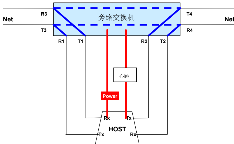
光路连接示意图
