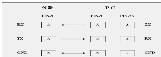
RS-232串口连接示意图
