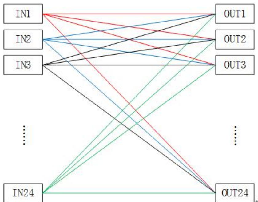
24×24 光开关内部光路示意图
